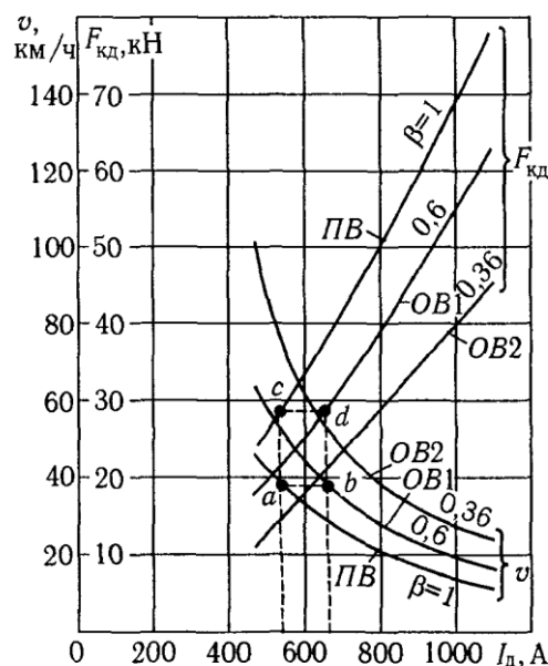
Рисунок 2.1 – Скоростные и электротяговые характеристики ТЭД ЭД118А
