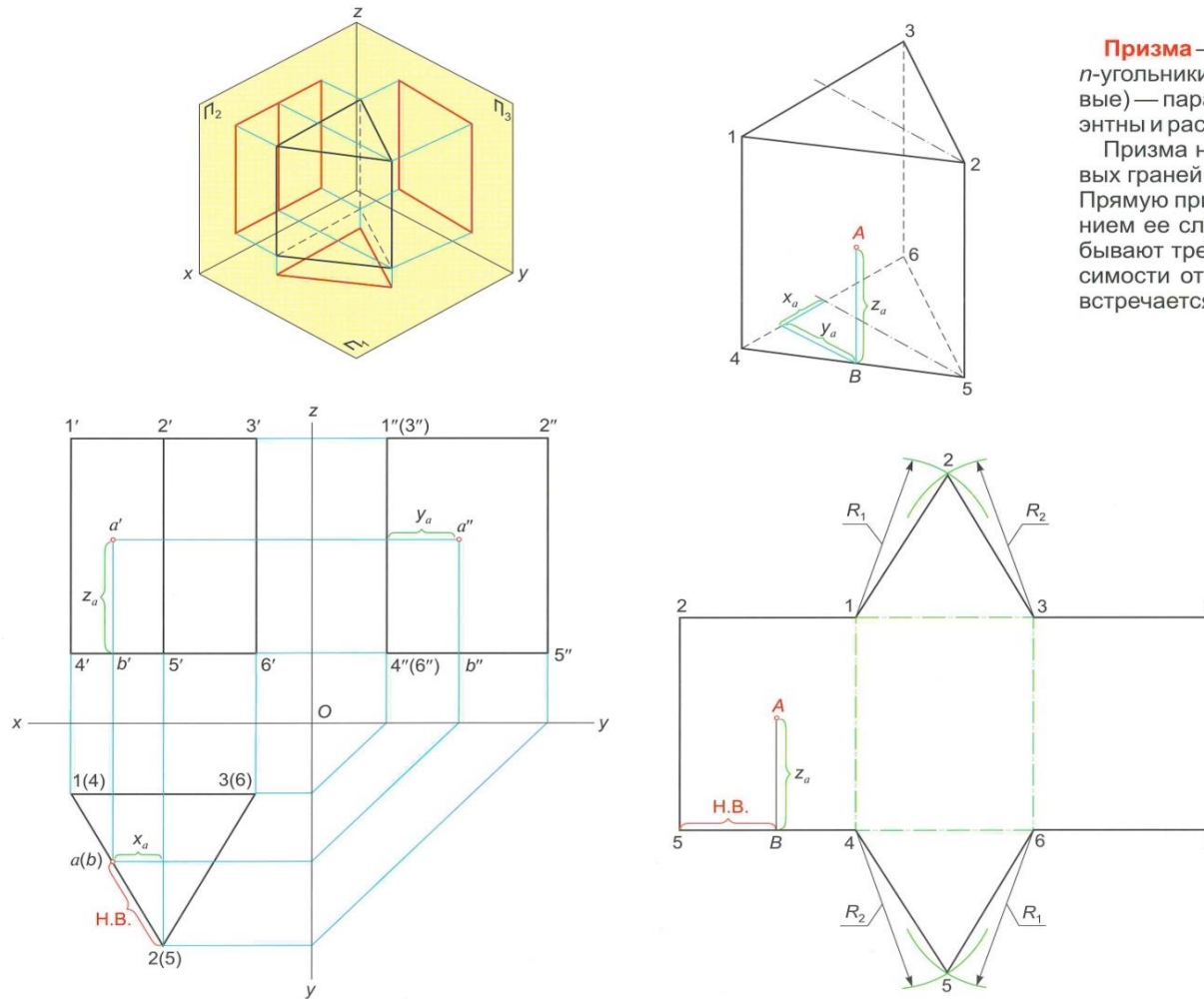
Рисунок 2 – Проекция трехгранной призмы
