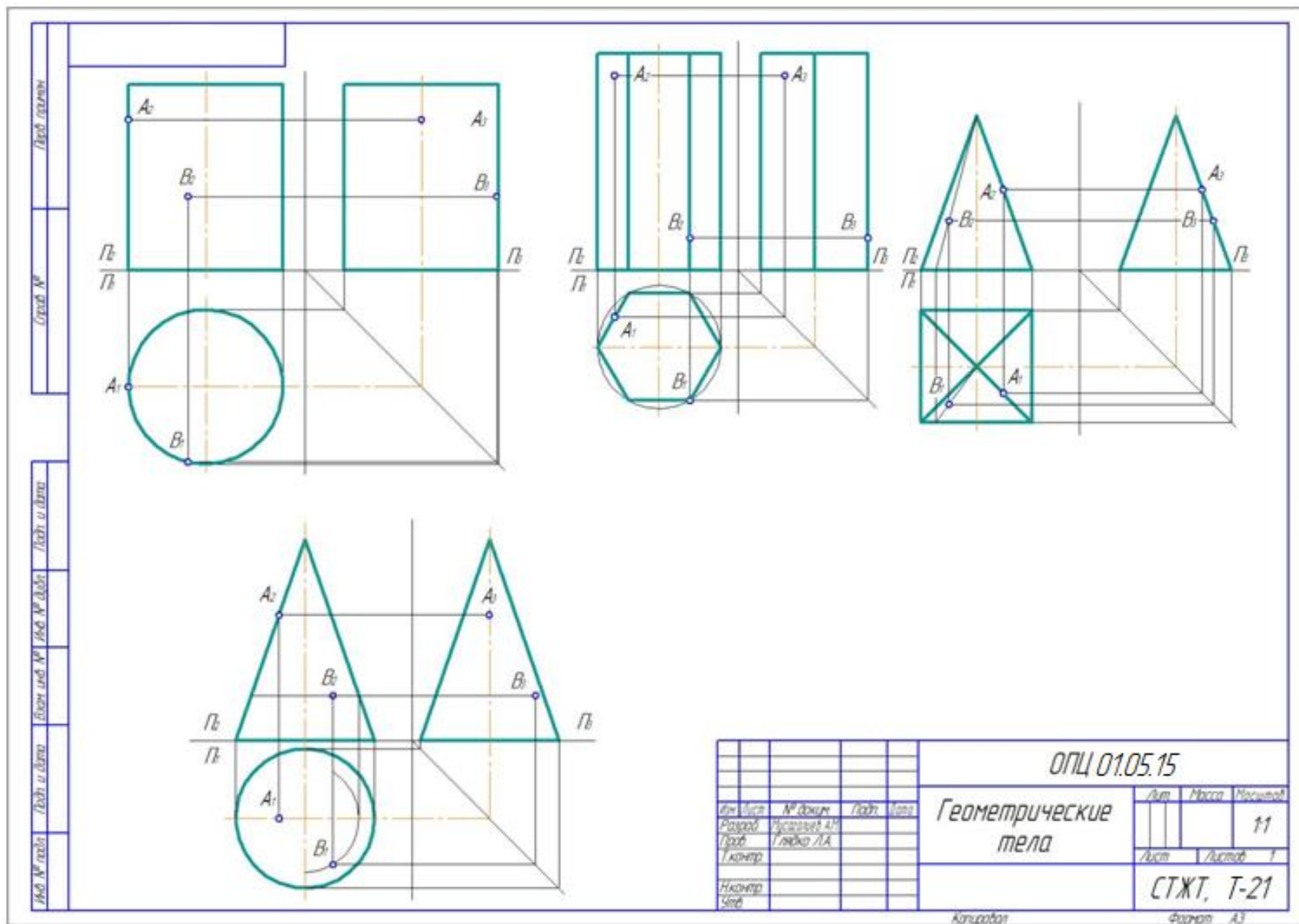
Рисунок 1 – Комплексный чертеж геометрических тел
