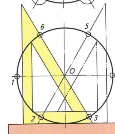
Рисунок 1 – Деление окружности на равные части
