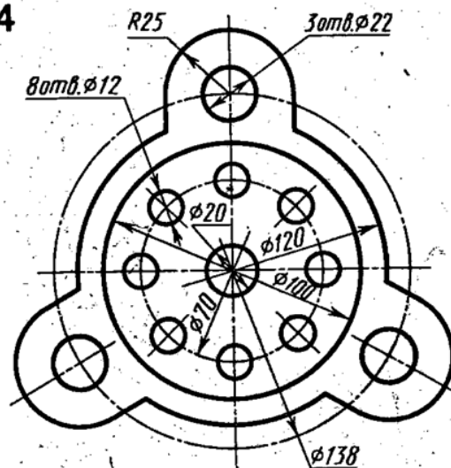
Фланец
