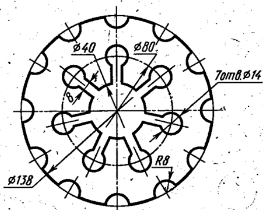
Прокладка
