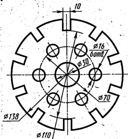
Прокладка
