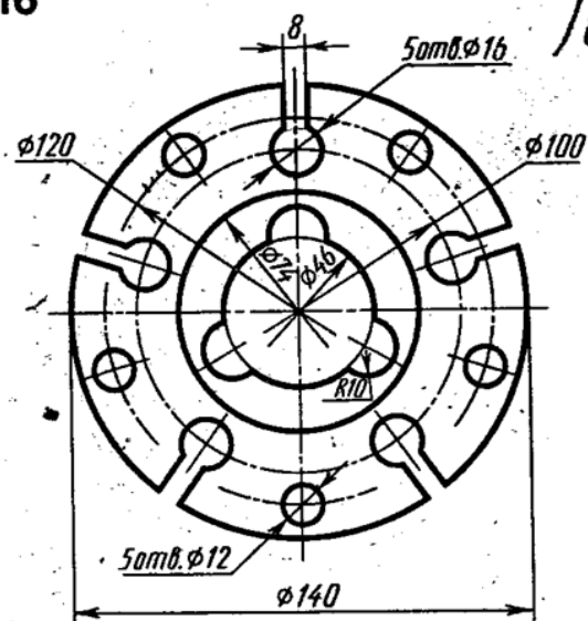
Прокладка
