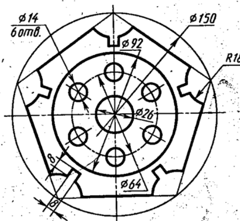
Крышка
