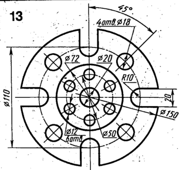
Фланец
