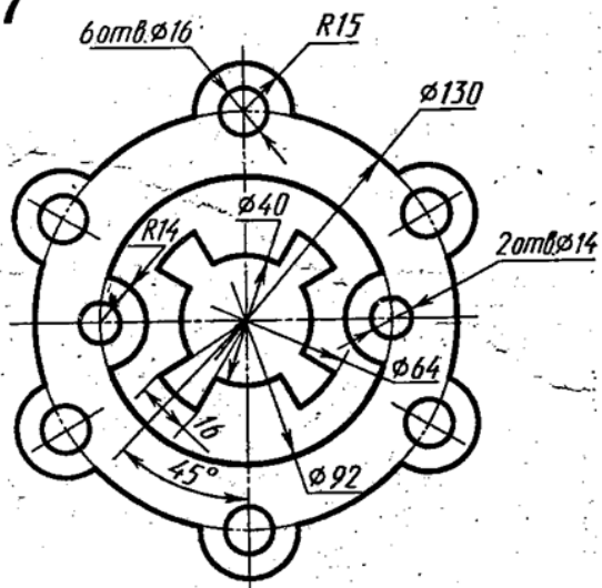
Пластина
