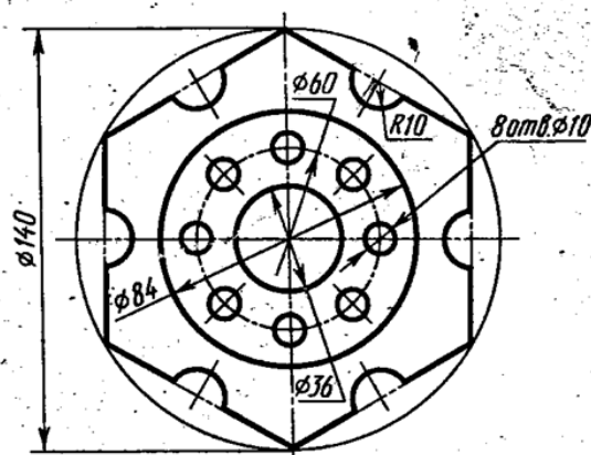
Пластина
