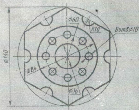
Пластина
