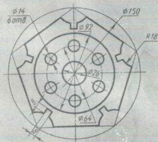
Крышка
