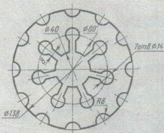
Прокладка
