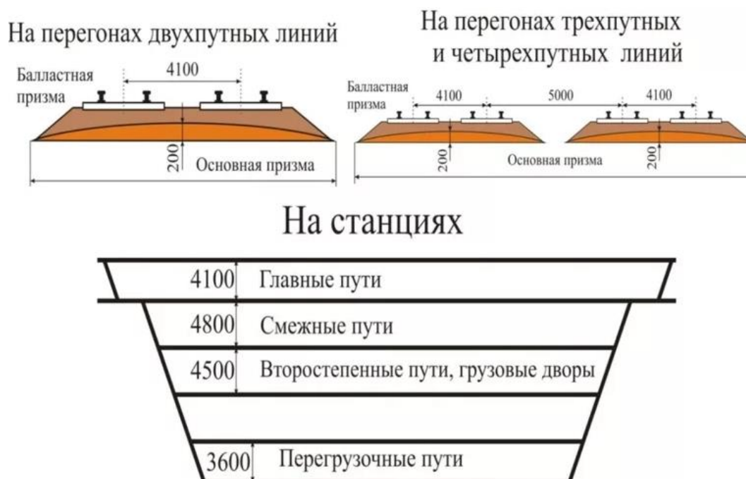
Рис. 2. Расстояние между осями путей
