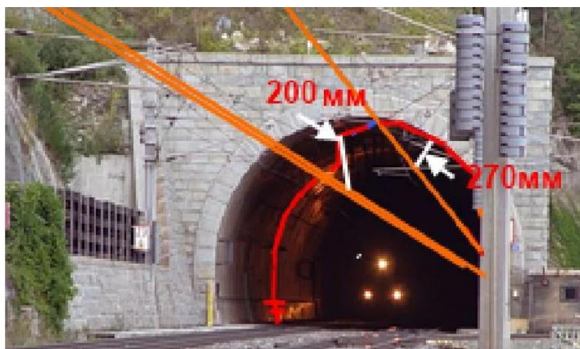
Рис. 13. Расстояние от токоведущих элементов токоприемника и частей контактной сети, находящихся под напряжением, до заземленных частей сооружений и железнодорожного подвижного состава в пределах искусственных сооружений
