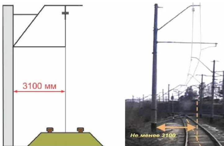
Рис. 13. Расстояние от оси крайнего железнодорожного пути до внутреннего края опор контактной сети на перегонах и железнодорожных станциях
