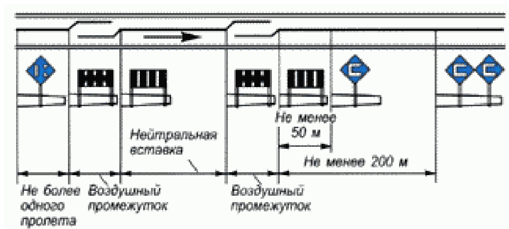
Рис. 163 (на железнодорожных путях общего пользования)
