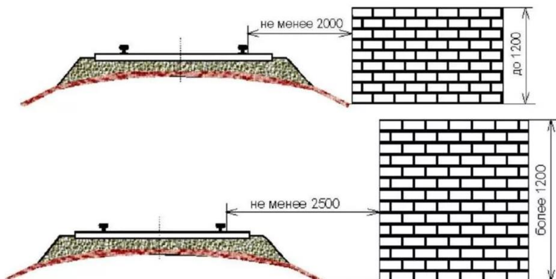
Рис. 4. Требования к грузам, выгруженным из вагонов или контейнеров либо подготовленным к погрузке
