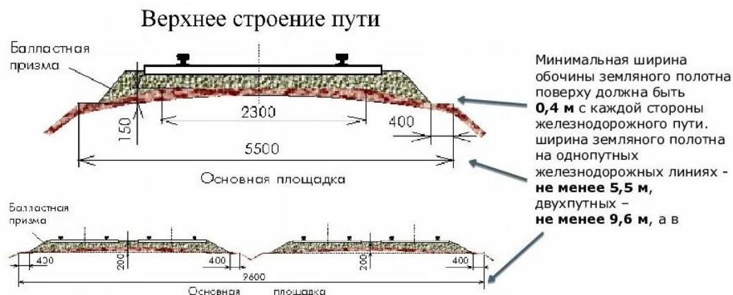
Рис. 8. Верхнее строение пути
