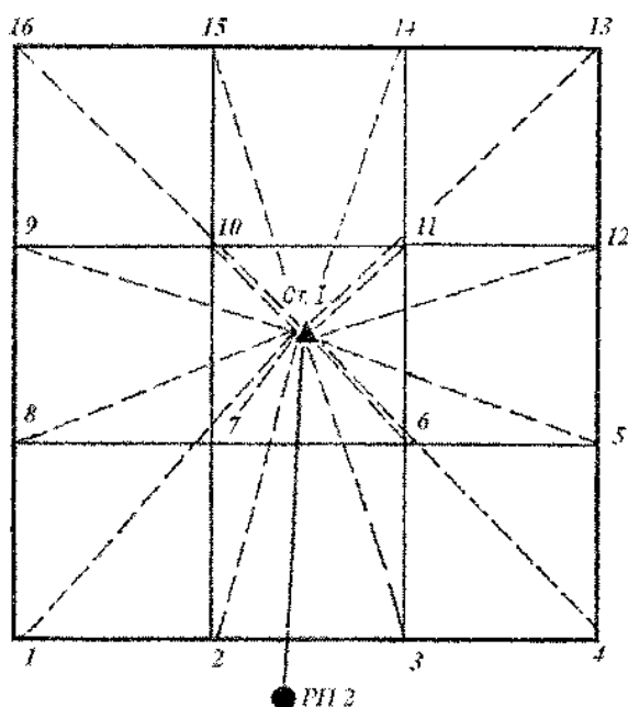
Рис. 11. Пример плана нивелируемой поверхности
