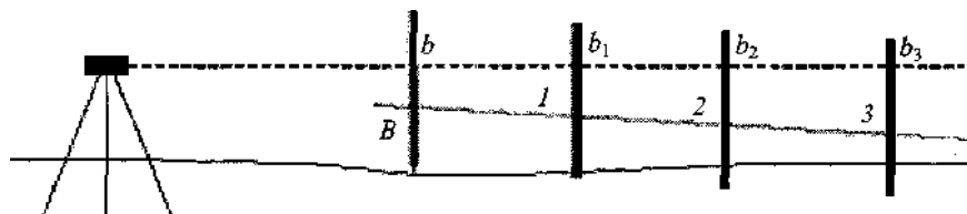
Рис. 5, а. Схема построения линии заданного уклона
