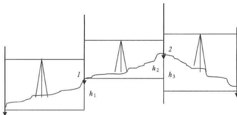
Рис. 7. Выполнение геометрического нивелирования
