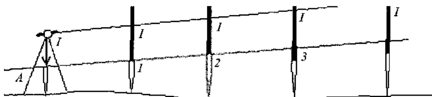
Рис. 5, 6. Схема построения наклонной линии
