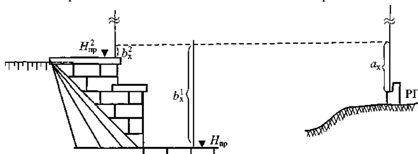
Рис. 4. Схема выноса проектных отметок
