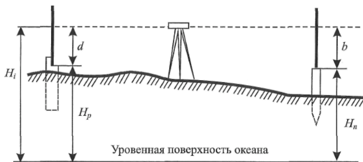
Рис. 3. Схема выноса в натуру проектной высоты В месте вынесения проектной высоты устанавливают рейку, опуская или поднимая ее
