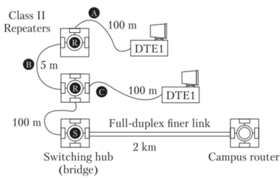
Рис. Л.28. Пример допустимой конфигурации сети Fast Ethernet
