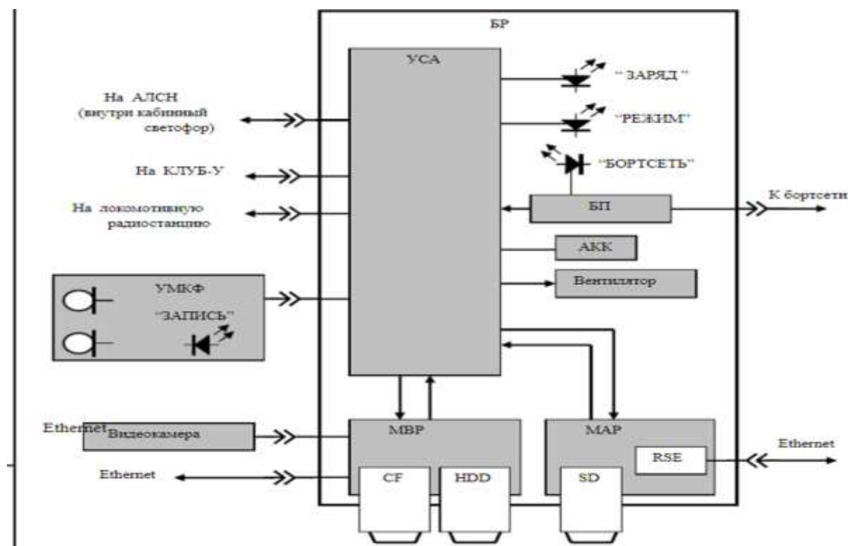
Рис. 5. Структура КВАРЦ
