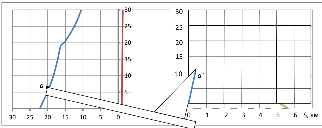
Рисунок 5.2 – Построение кривой скорости в функции пути при движении по горизонтальному прямолинейному пути при средней скорости v=5 км/ч
