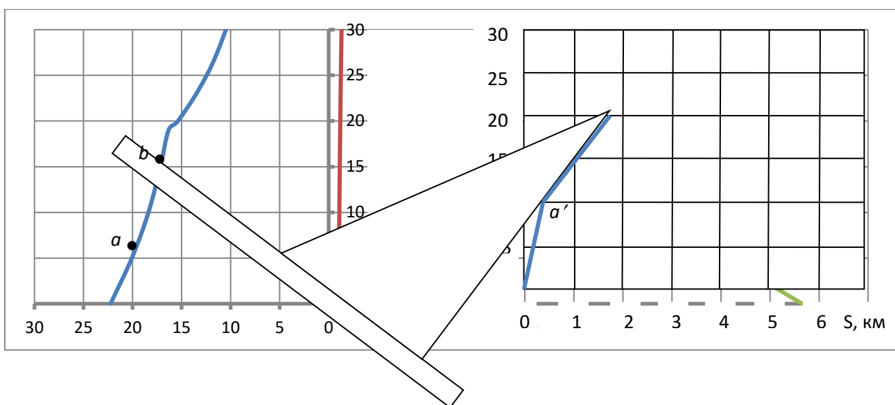
Рисунок 5.3 – Построение кривой скорости в функции пути при движении по горизонтальному прямолинейному пути при средней скорости v=15 км/ч
