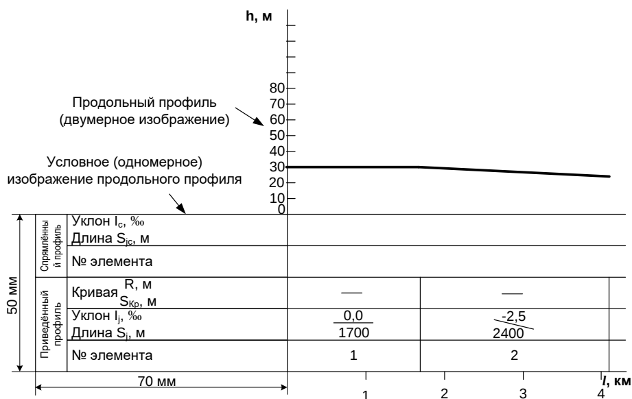
Рисунок 4.1 – Пример оформления продольного профиля пути
