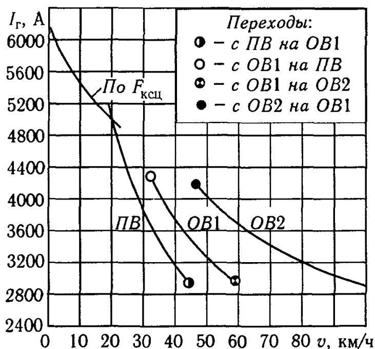
Рисунок 7.1 – Зависимость тока генератора тепловоза 2ТЭ116 от скорости
