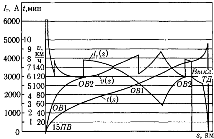
Рисунок 7.2 – Построение кривой тока генератора тепловоза
