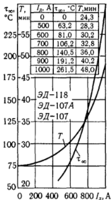
Рисунок 8.1 – Тепловые характеристики тягового электродвигателя ЭД-118 тепловоза 2ТЭ116
