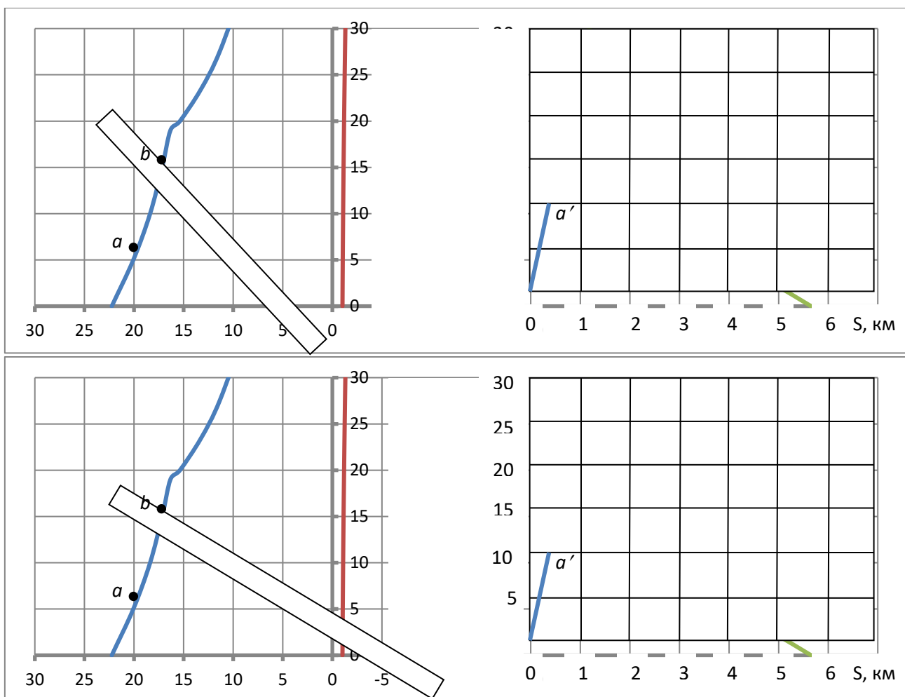
Рисунок 5.4 – Построение кривой скорости в функции пути при движении на подъёме или на спуске
