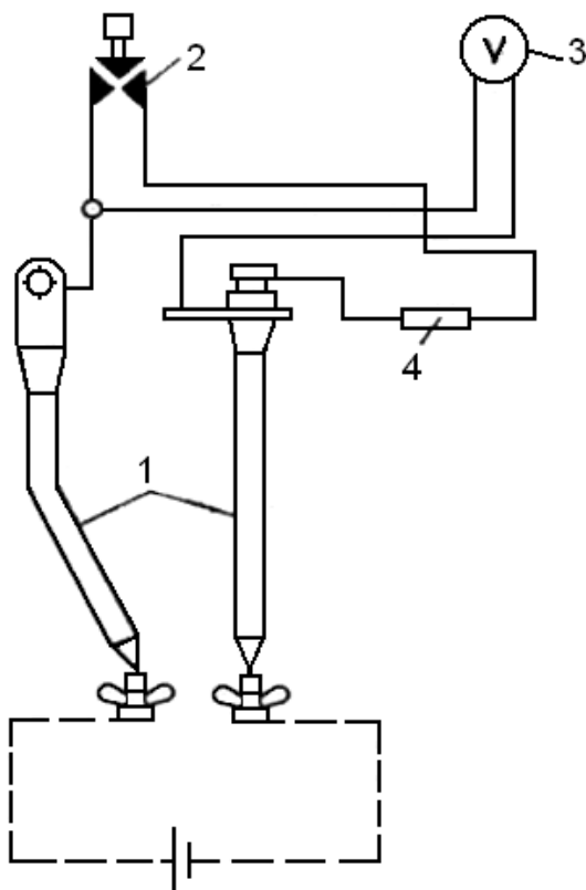
Рисунок 11.3 - Схема включения нагрузочной вилки:
