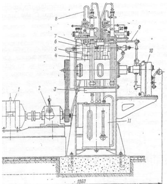
Рисунок 5.1 – Стенд для испытания топливных насосов типа А77:
