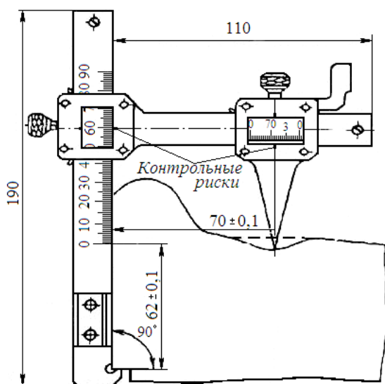
Рисунок 2.4 - Измерение толщины бандажа
