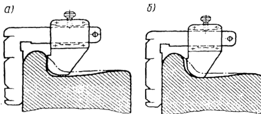
Рисунок 2.6 - Выявление вертикального подреза гребня:
