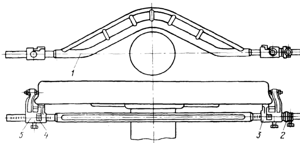
Рисунок 2.9 - Бандажный штангенциркуль:
