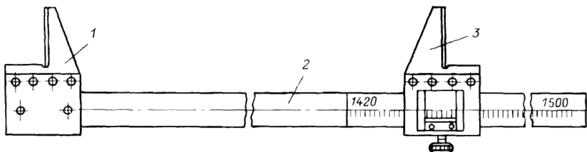
Рисунок 2.8 - Межбандажный штангенциркуль:
